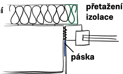
řez ostěním
