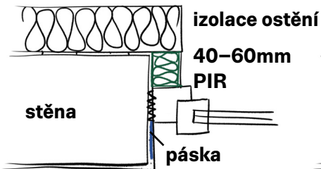
řez ostěním
